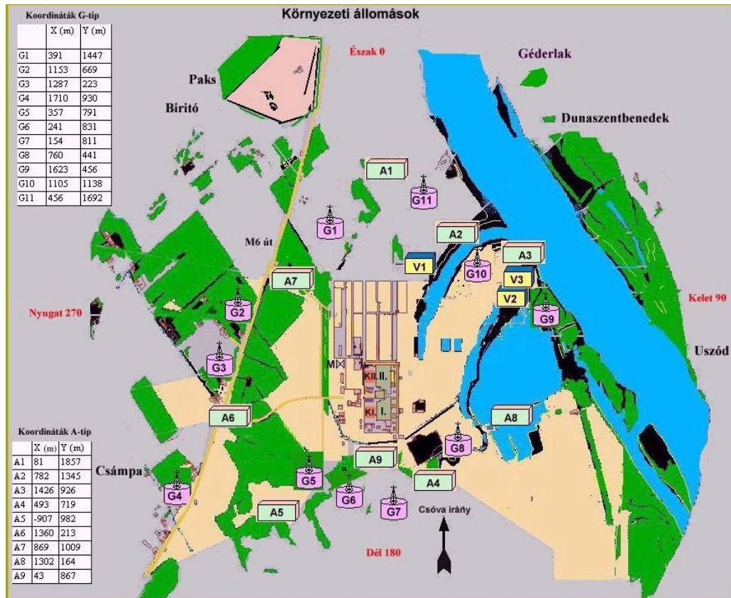
1.1.a ábra Az atomerőmű környezeti elhelyezkedése az üzemi monitorozó hálózattal.
