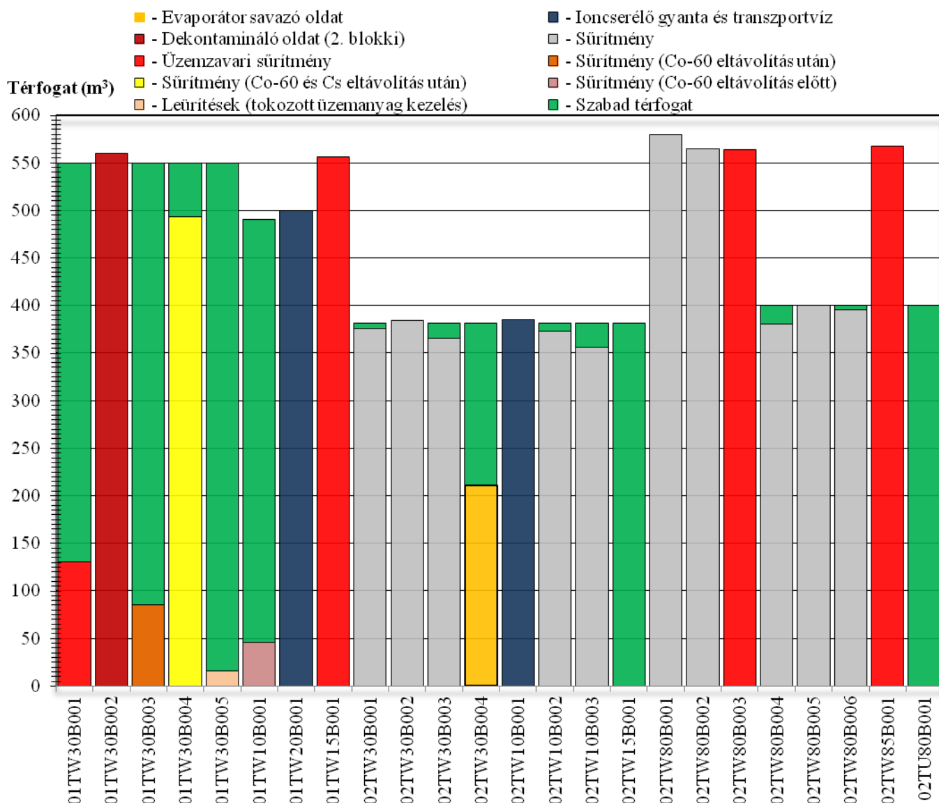
3.1. ábra. A folyékony hulladéktároló tartályok töltöttsége (2013. decemberi állapot).
