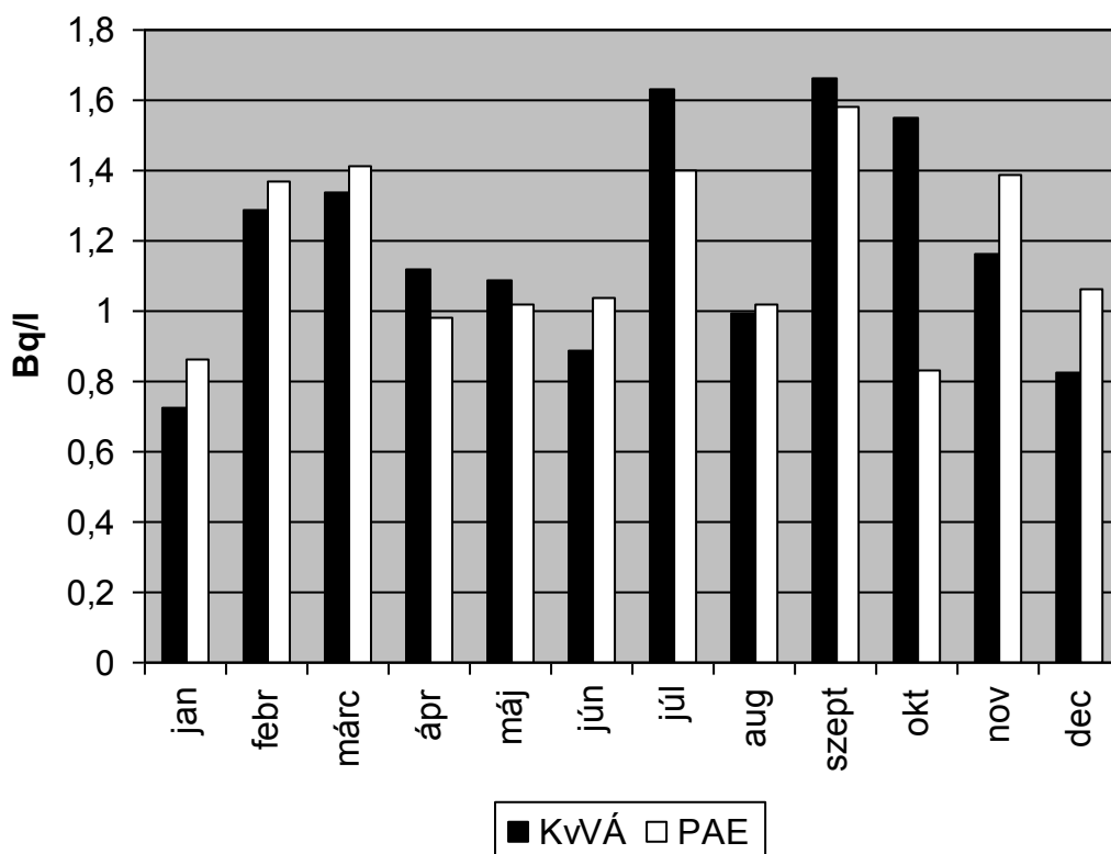
2.4.c. ábra. A szennyvíz csatorna (V3) összes-béta aktivitáskonzentrációjának havi átlagértékei. Figure 2.4.c. Monthly gross beta activity concentration in the waste water channel (KVvÁ: measured by SEW; PAE: measured by NPP).
